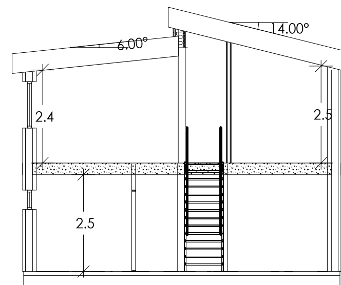
Sektion
